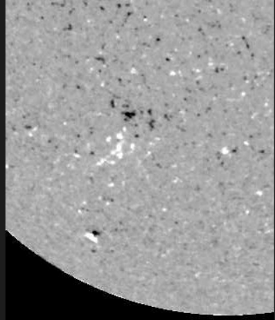
Magnetogram (Tuesday)
